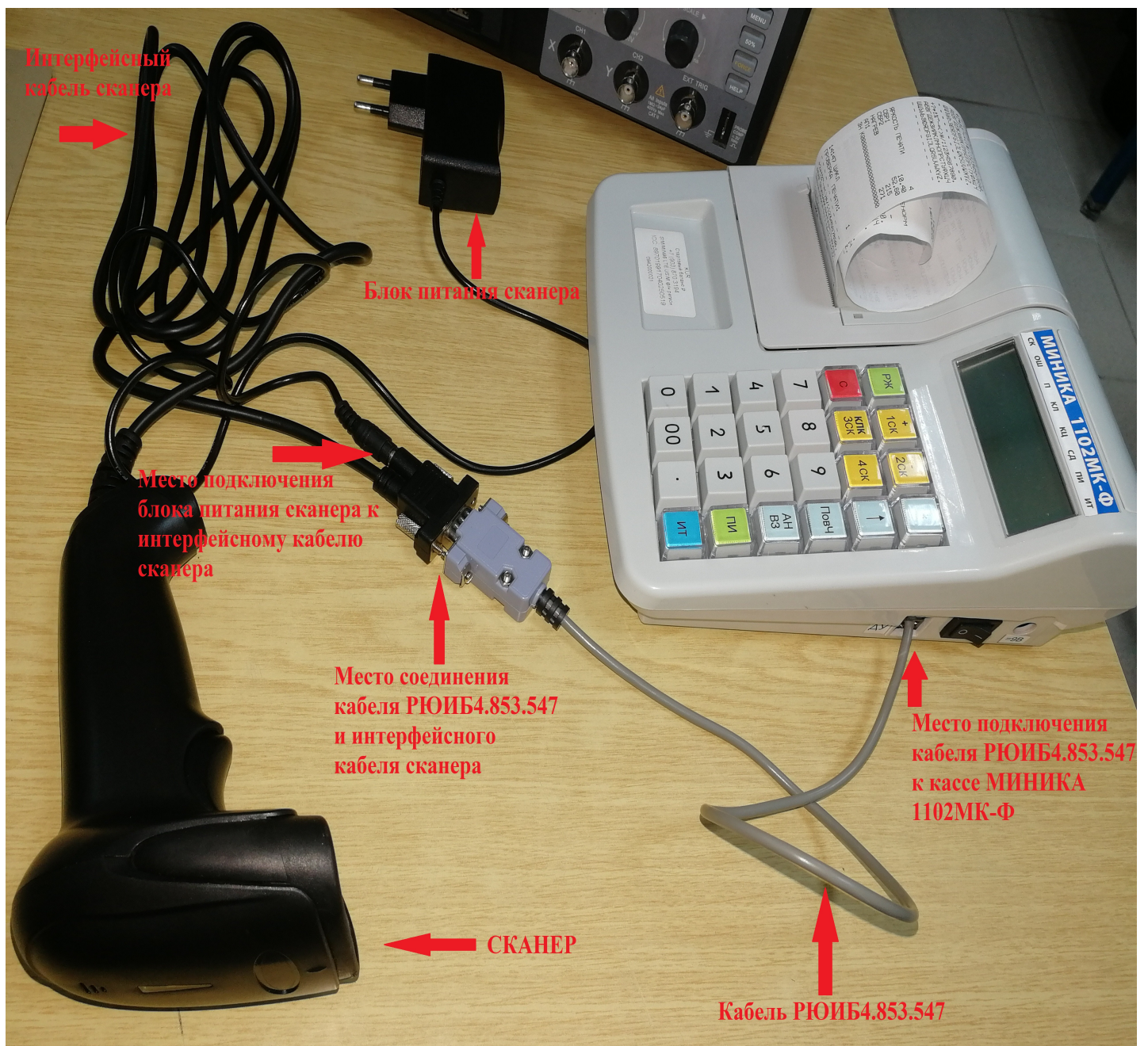
Рис.1 Подключение сканера к кассе МИНИКА 1102МК-Ф
